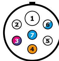
Steckdose 7-polig
