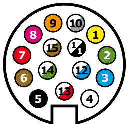
Steckdose 15-polig
