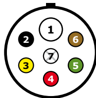
Steckdose 7-polig
